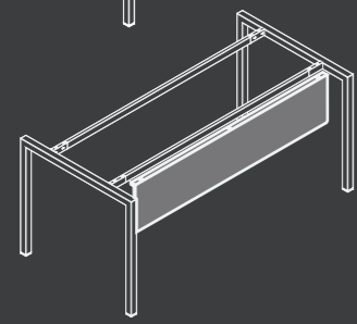
Frontal Panel Avental Frontal Voile Fond Faldón Devant
